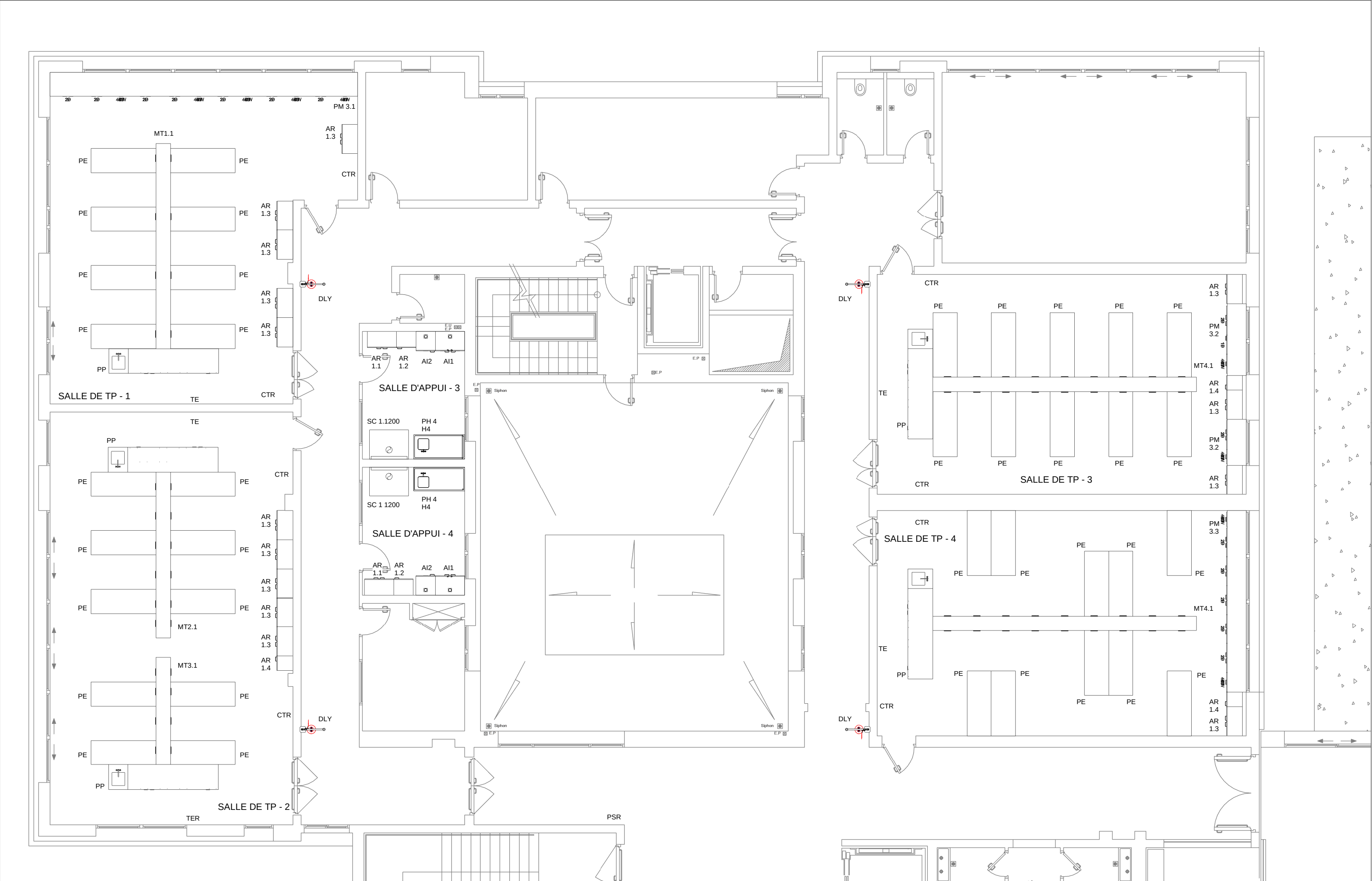
BAT-B 2 éme 1 : 100
